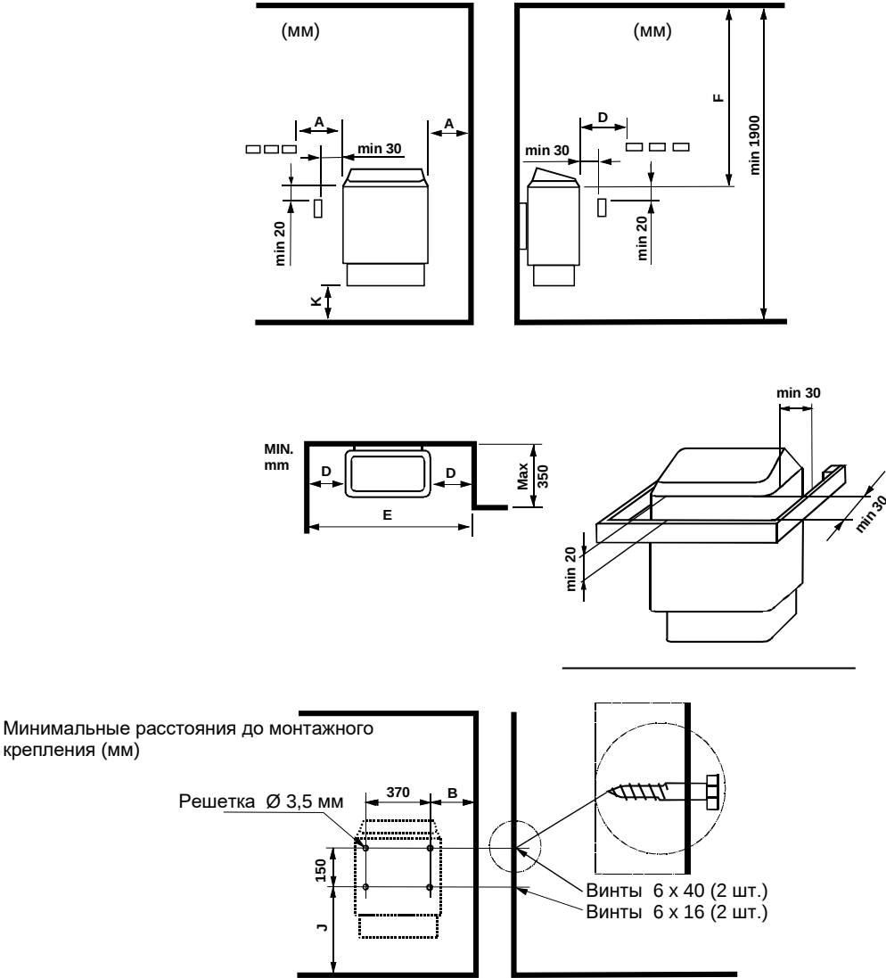
Рис. 2 Безопасные расстояния
